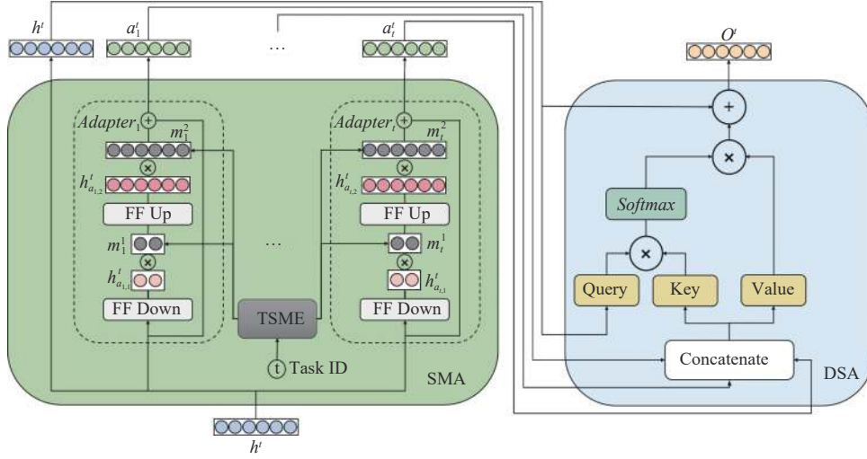
图3 SMA 模块和 DSA 模块
