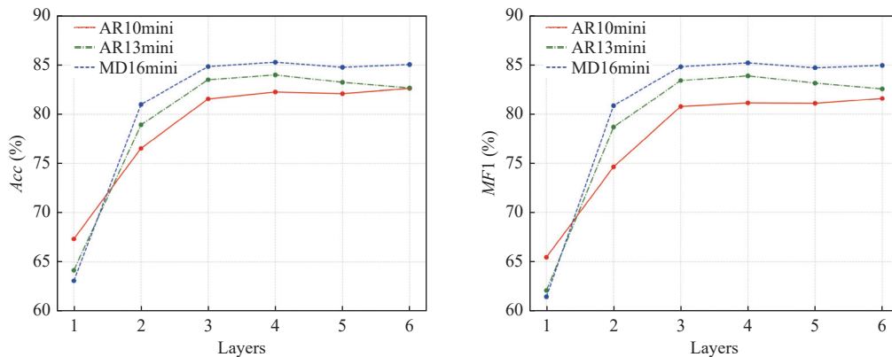
图 4 关于 Transformer layer 数的对比实验结果
