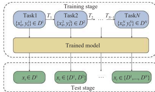
图1 针对连续情感分析任务的持续学习过程
