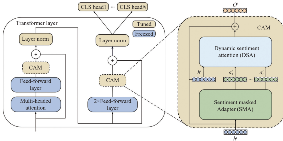
图2 本文使用的 Transformer layer 和 CAM 模型总体结构
